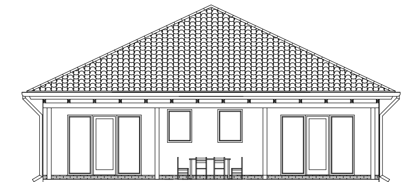
POHLED BOČNÍ - LEVÝ
