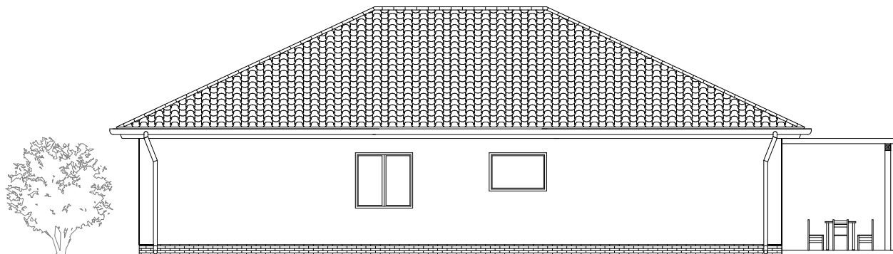
POHLED ZADNÍ
