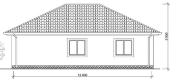
POHLED BOČNÍ - PRAVÝ
