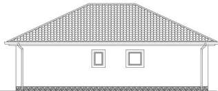
POHLED BOČNÍ - LEVÝ
